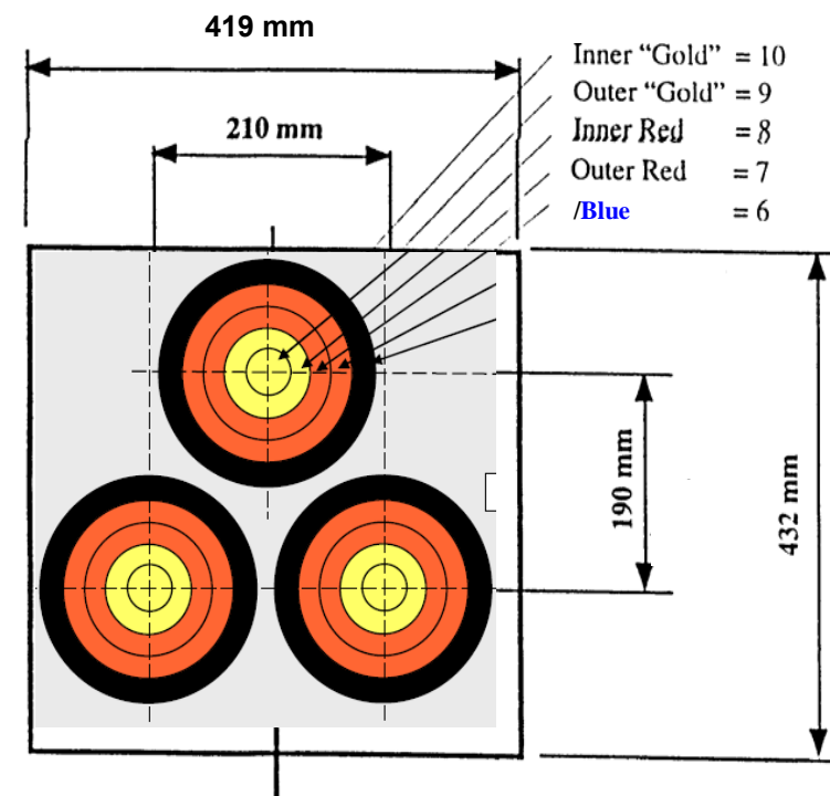
Рис. 317.1.1 Тройная мишень диаметром 60см:
