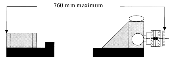
Рис. 326-2 Ограничение на длину прицельной линии
