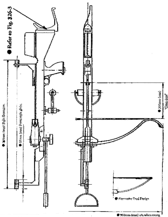
Рис. 326-1 Параметры Арбалета (См. ст. 326.5.1)
